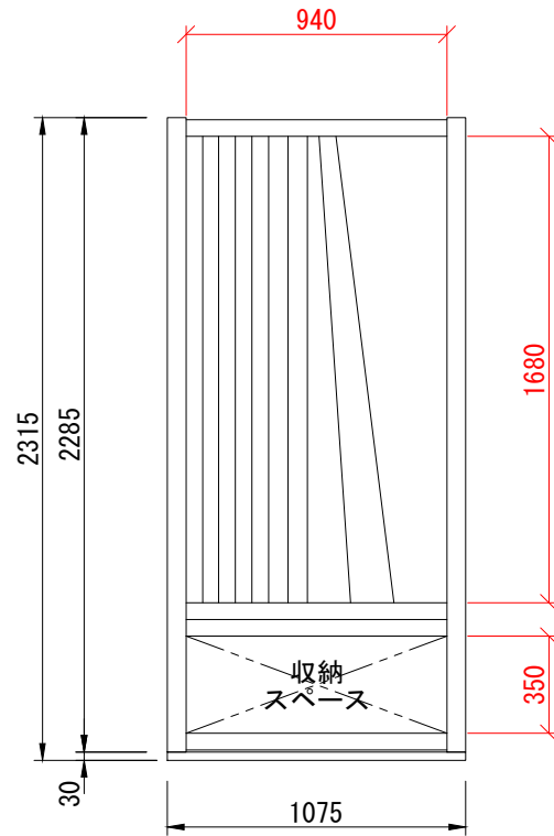
正面
