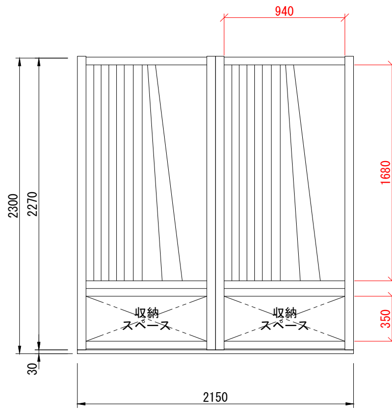
正面
