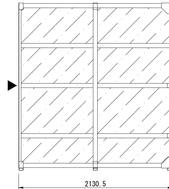
側面
