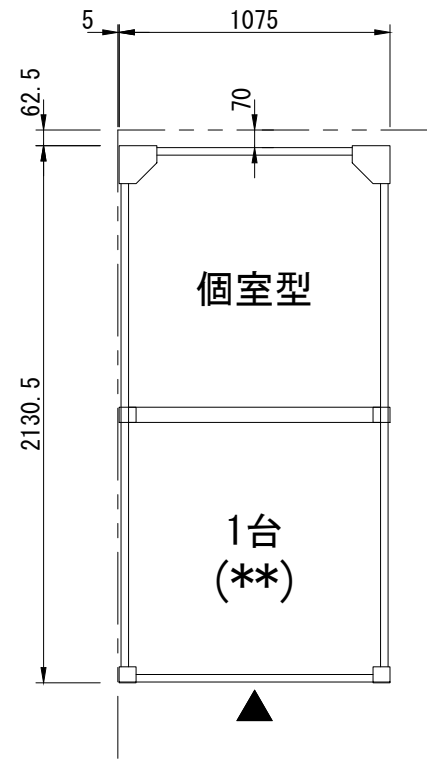
平面
